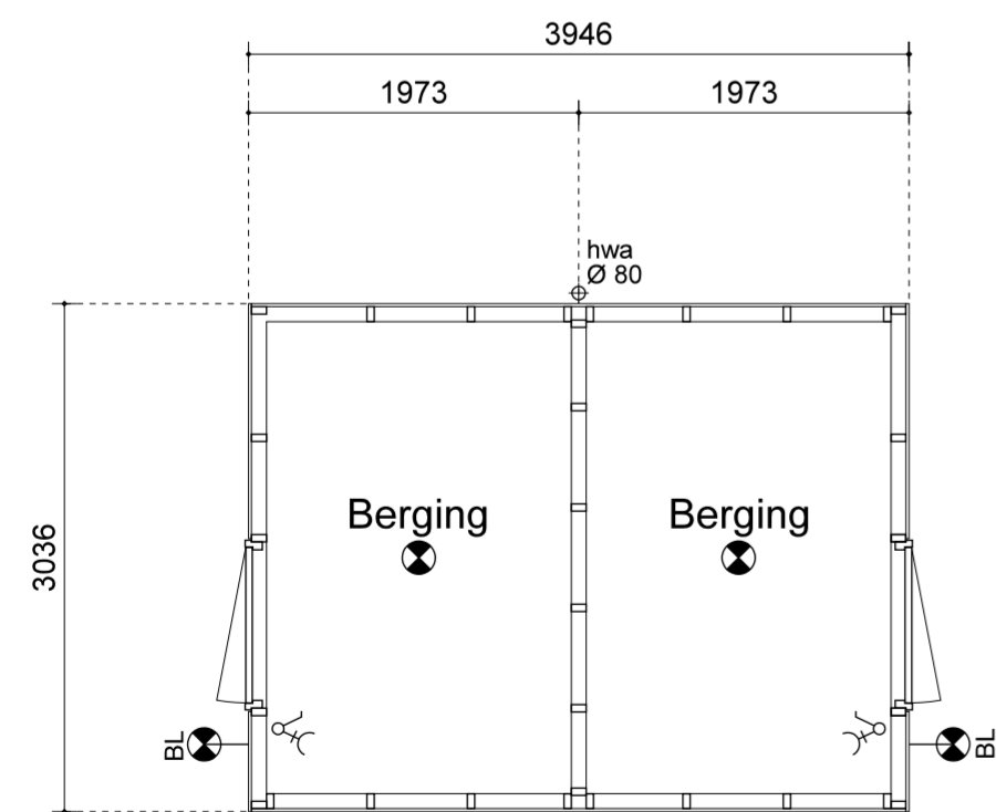
PLATTEGROND
