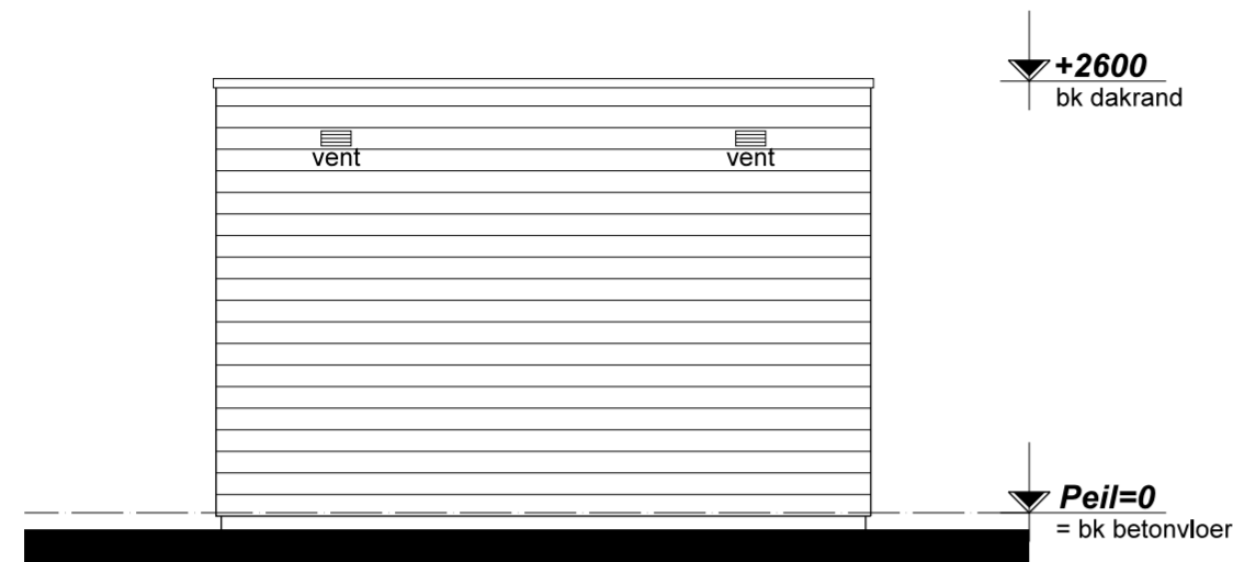
VOORGEVEL
