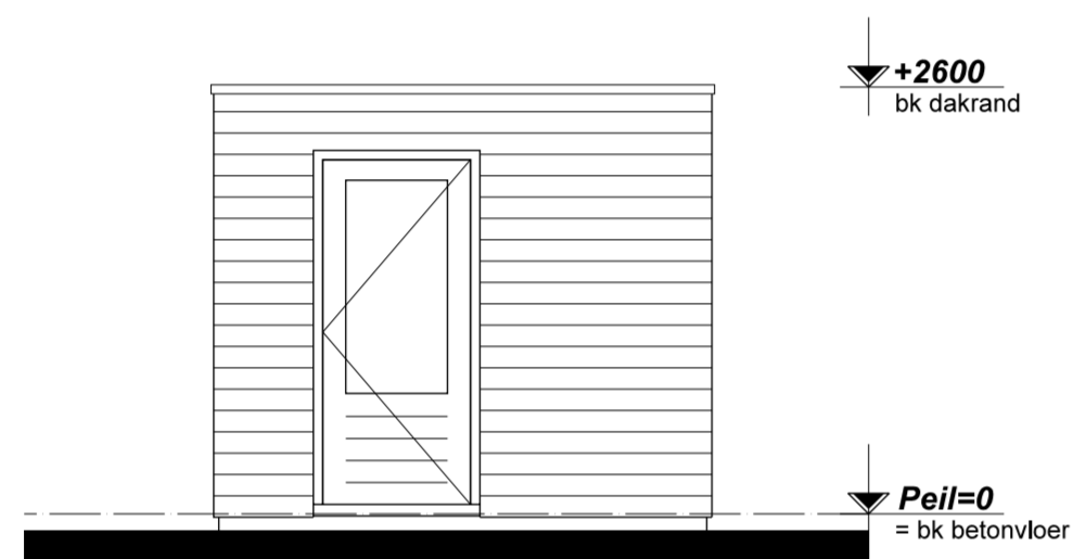
RECHTERZIJGEVEL
