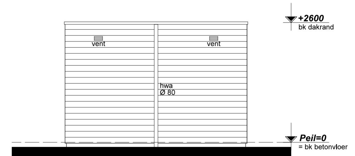
ACHTERGEVEL
