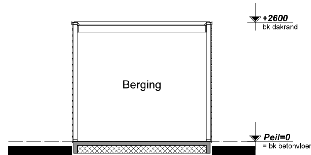
DOORSNEDE
